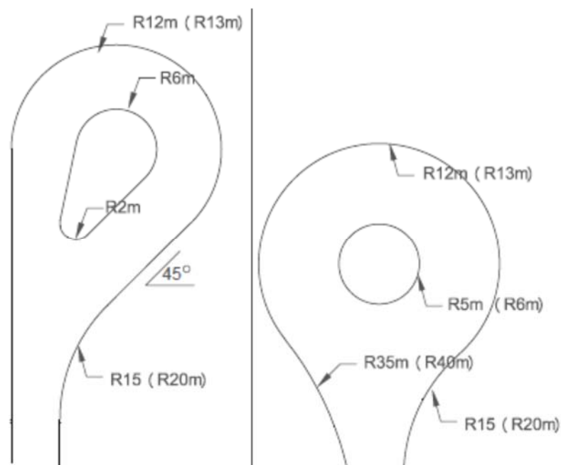
Figur 16. Snuplasser reguleres med bredde som tilsvarer veiens kjørebane og sideareal og opparbeides med asfaltbredder som for kjørevei. Tall i parentes gjelder samleveier.
